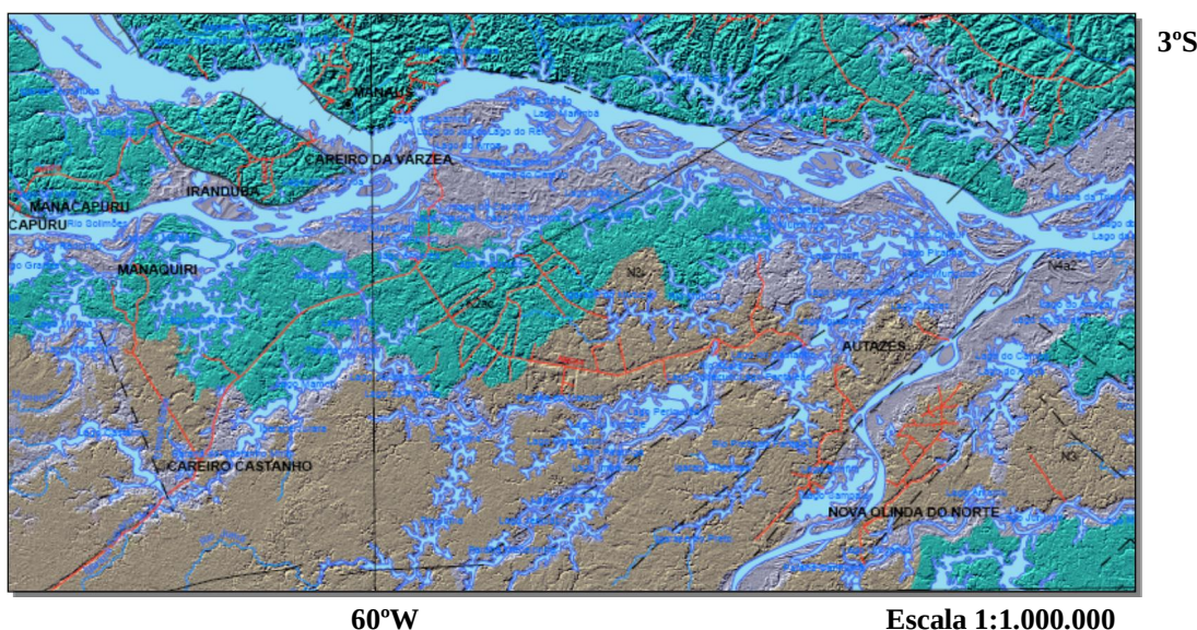
Figura 7: Aspectos geológicos da área da pesquisa em mosaico completo.
