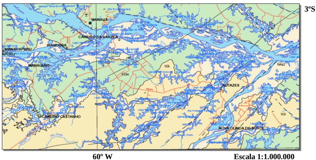
Figura 6: Aspectos geológicos da área da pesquisa.
